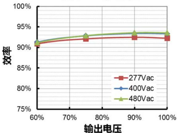
ESM-240S150Bx( I_o=1050mA ) 效率 vs. 输出电压
