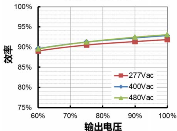
ESM-240S150Bx( I_o=1500mA ) 效率 vs. 输出电压
