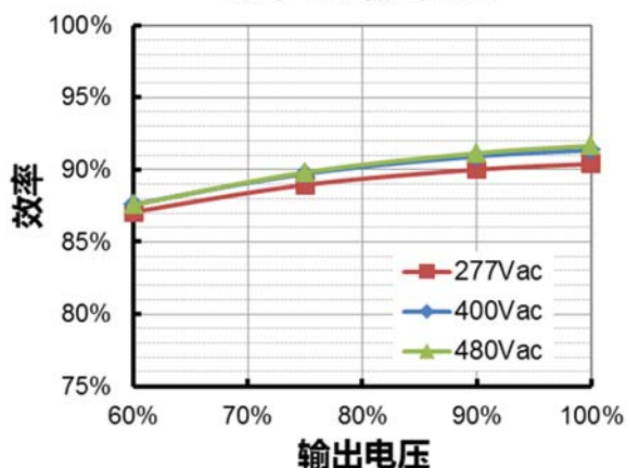
ESM-240S350Bx( I_o=3500mA ) 效率 vs. 输出电压
