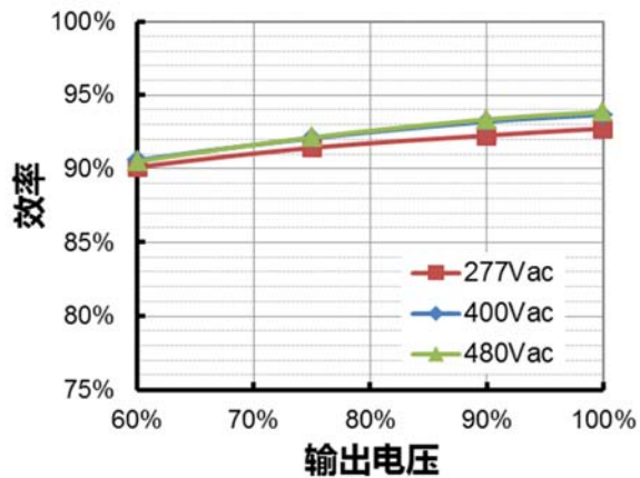
ESM-240S105Bx( I_o=1050mA ) 效率 vs. 输出电压
