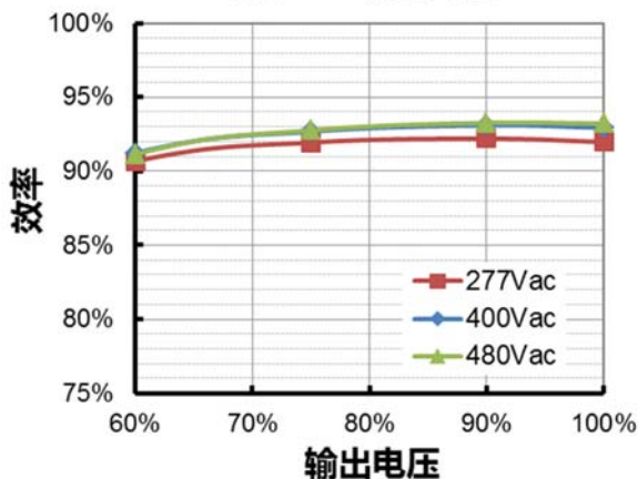
ESM-240S350Bx( I_o=2150mA ) 效率 vs. 输出电压
