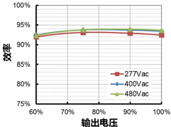
ESM-240S105Bx( I_o=700mA ) 效率 vs. 输出电压
