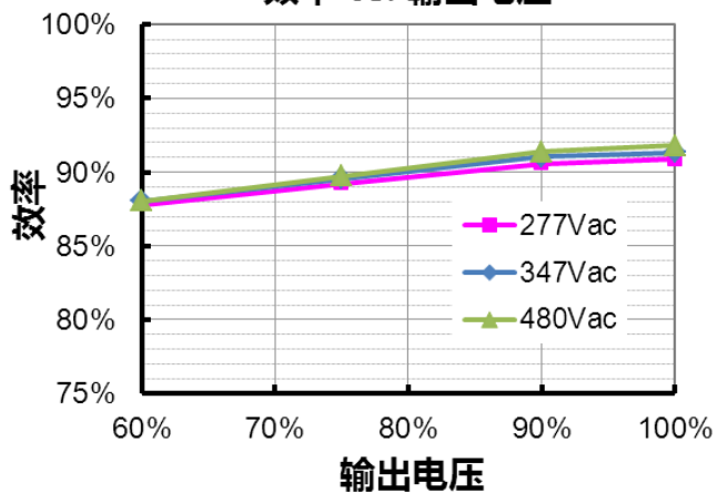
ESD-480S10ADT (Io=10000mA) 效率 vs. 输出电压
