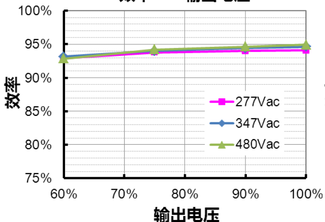
ESD-480S140DT (Io=1050mA) 效率 vs. 输出电压
