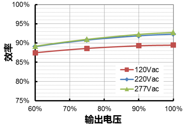
EUK-240S150DT(TT)( I_o=1500mA ) 效率 vs. 输出电压
