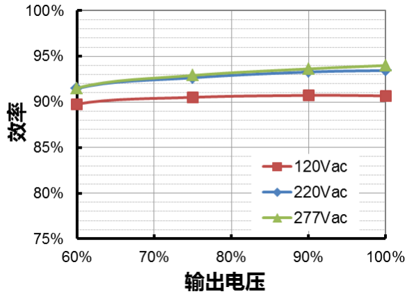
EUK-240S150DT(TT)( I_o=1050mA ) 效率 vs. 输出电压
