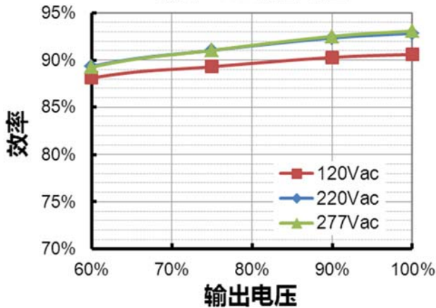
EUD-096S105BTA (Io=700mA) 效率 vs. 输出电压
