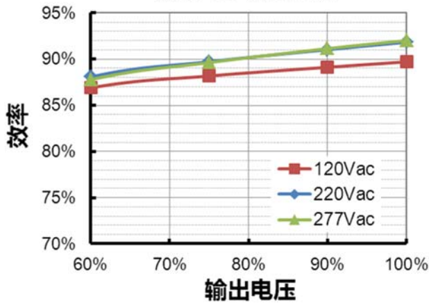
EUD-096S070BTA (Io=450mA) 效率 vs. 输出电压
