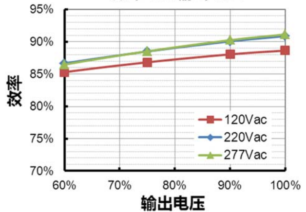
EUD-096S105BTA (Io=1050mA) 效率 vs. 输出电压
