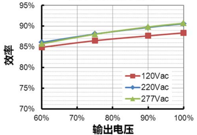
EUD-096S070BTA (Io=700mA) 效率 vs. 输出电压
